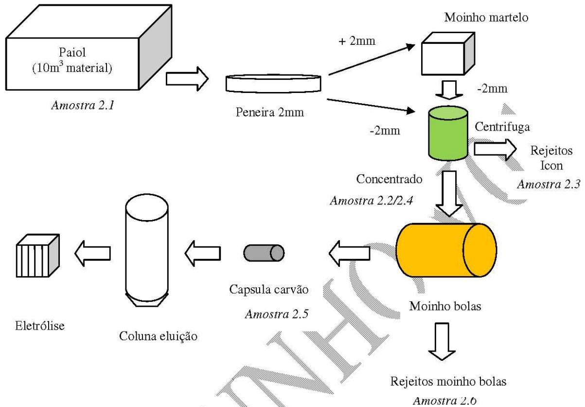
Figura 3 Fluxograma do processo da planta piloto
